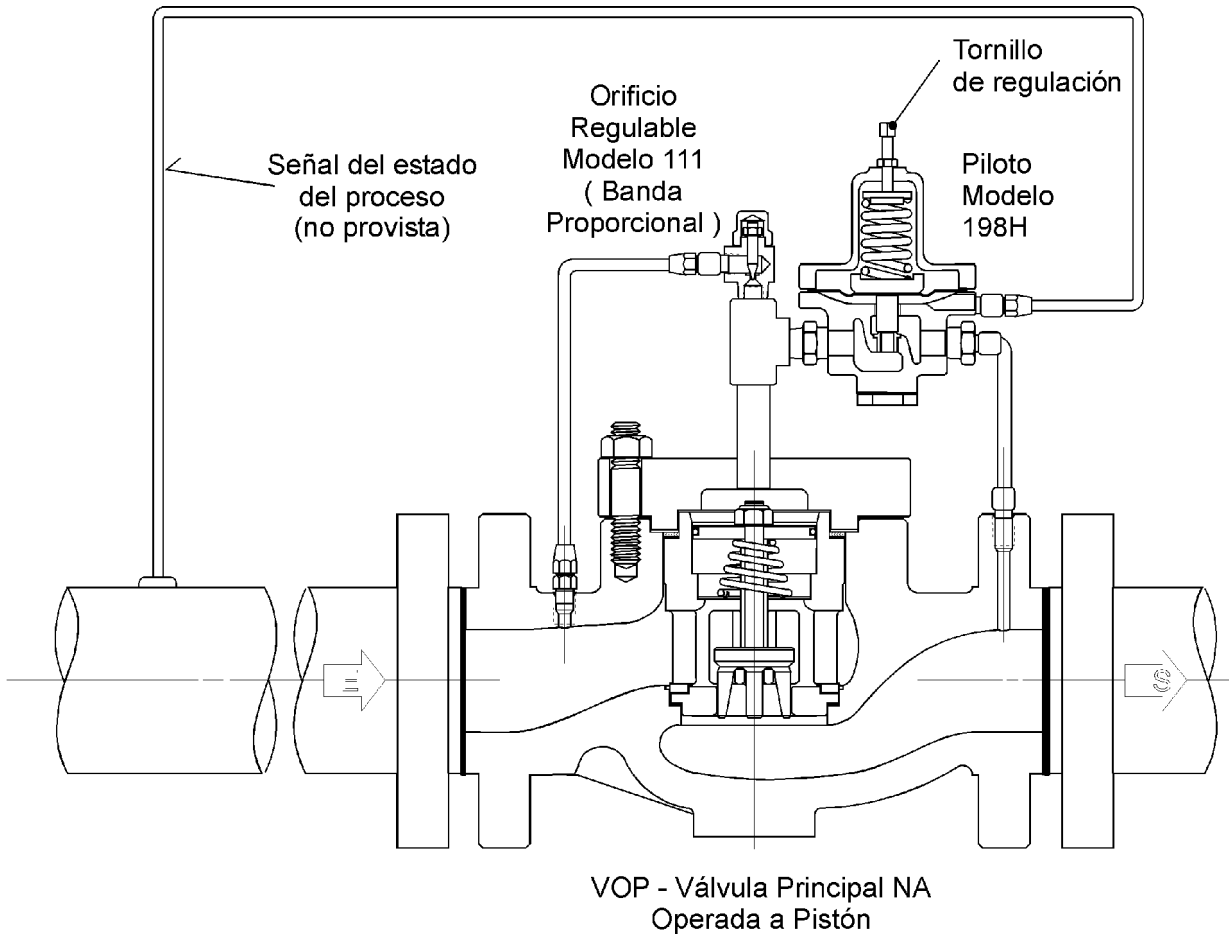
Fig.1.- Conexionado - Funcionamiento
