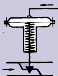
FIG. 7 657R (NA) - Normal Abierta - Aire a cerrar - Resorte abre - Flujo a abrir
