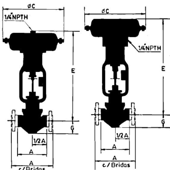
Fig. 5 - 657R (NA o NC)
