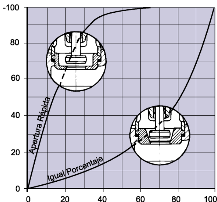
Fig. 4 - Cuerpo "R". Curvas de característica Inherente
