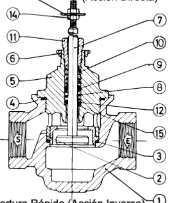
Fig. 16: Apertura Rápida (Acción Inversa)
