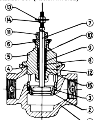
Fig. 15: Igual porcentaje (Acción Directa)
