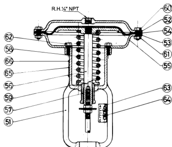
Fig. 13: Actuador 657 (Acción Directa)
