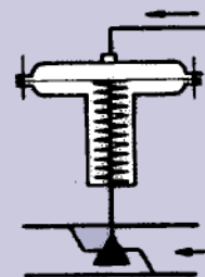
FIG. 9 667R (NC) - Normal Cerrada - Aire a abrir - Resorte cierra - Flujo a abrir - Solo orificios 16 a 35
